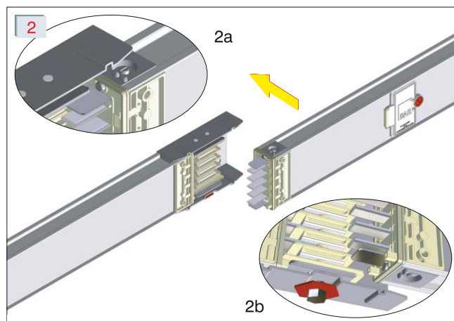
Шинопровод без блочного соединения монтируется таким образом, чтобы штыри на конце секции вошли в отверстия на стыке блока. (2a) Проследите за тем, чтобы пластиковые штыри, расположенные на конце секции были на стороне гайки со срезом. (2б)
