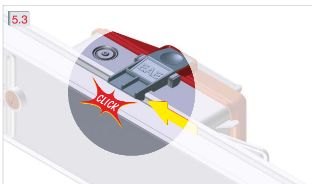
Убедитесь в том, что коробка прочно зафиксирована на корпусе шинопровода.
